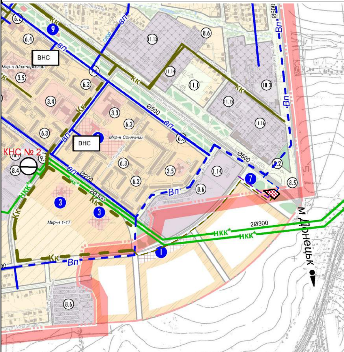
Викопіювання з генерального плану м. Покровськ (схема інженерного обладнання території (водопостачання, каналізація))
